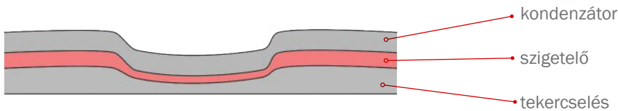
Shopguard címke keresztmetszete
